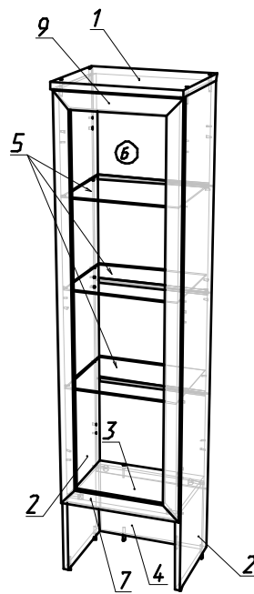
Рис.1 Схема сборки
